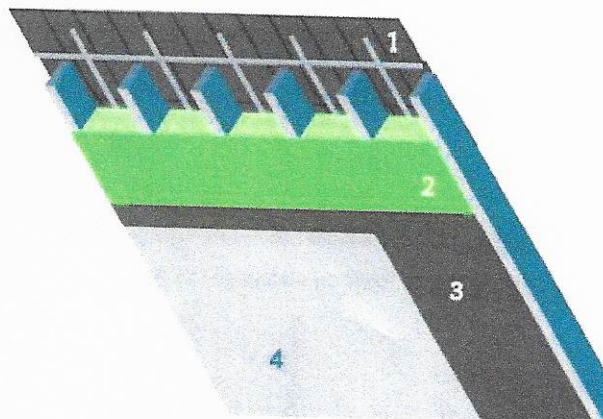
1. Onderdak | 2. Isolatatie | 3. Dampscherm | 4. binnenaafwerking
