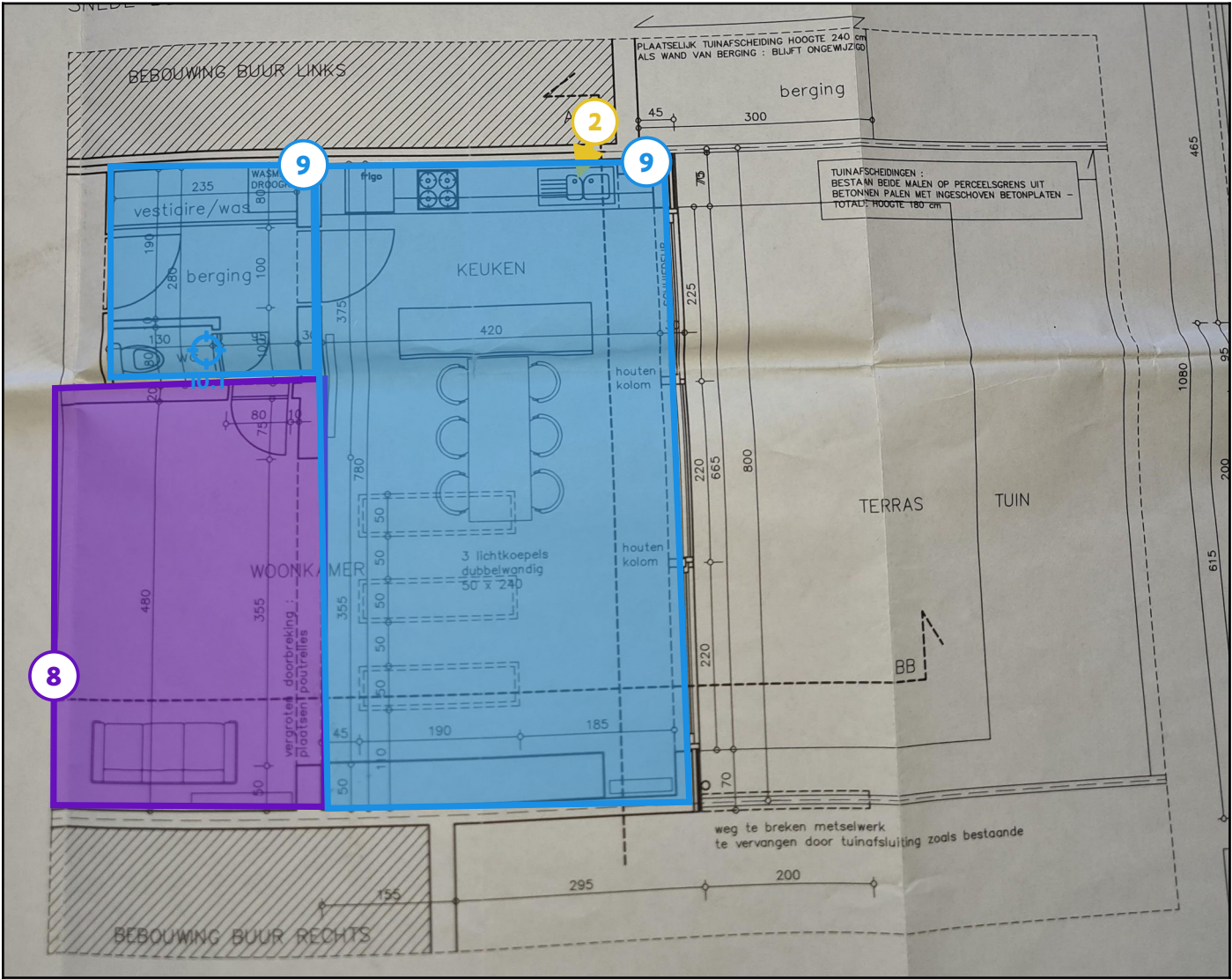
Legende van plan 1.3: Grondplan gelijkvloers nieuwe deel
