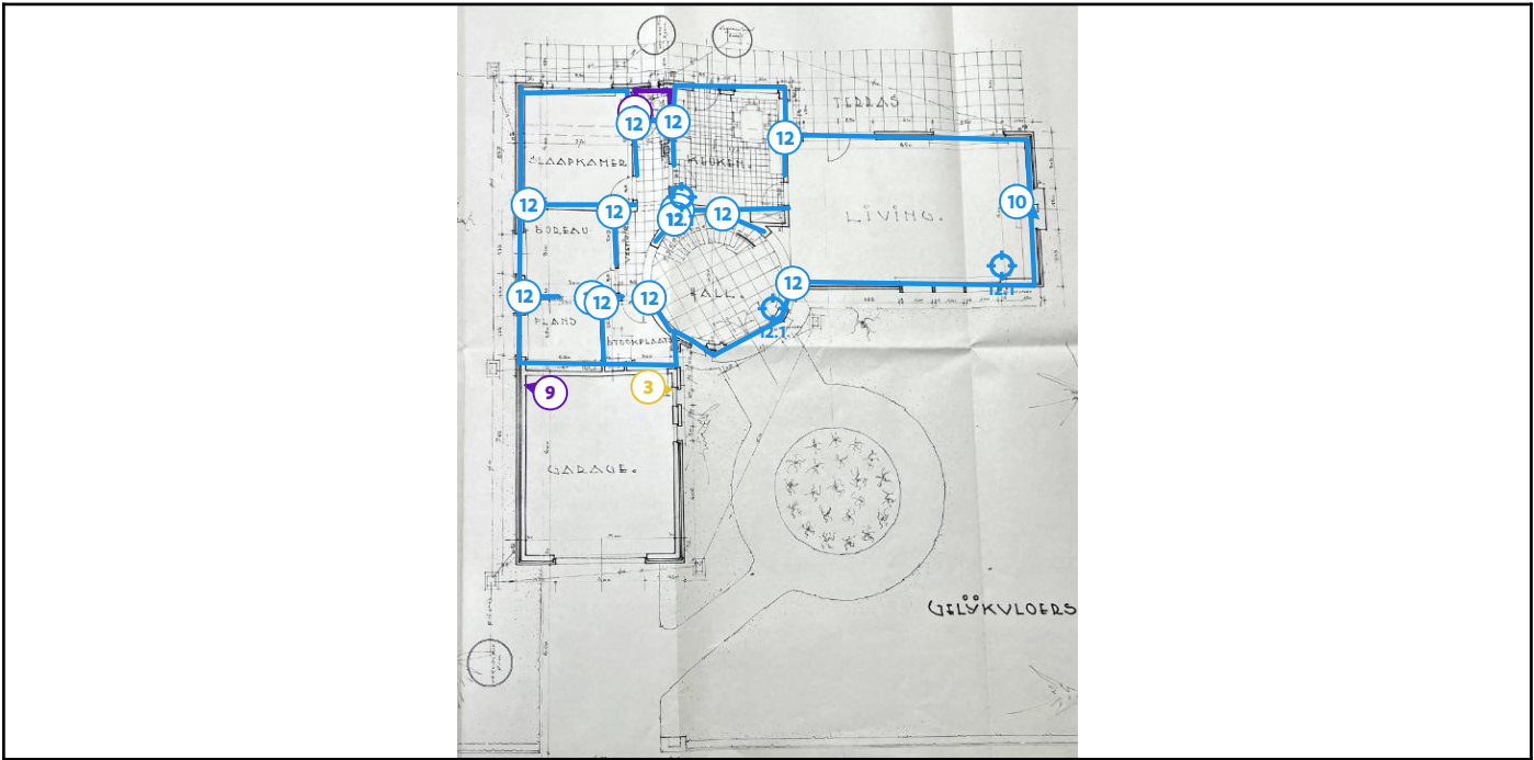
Legende van plan 3.3: Plan gelijkvloers
