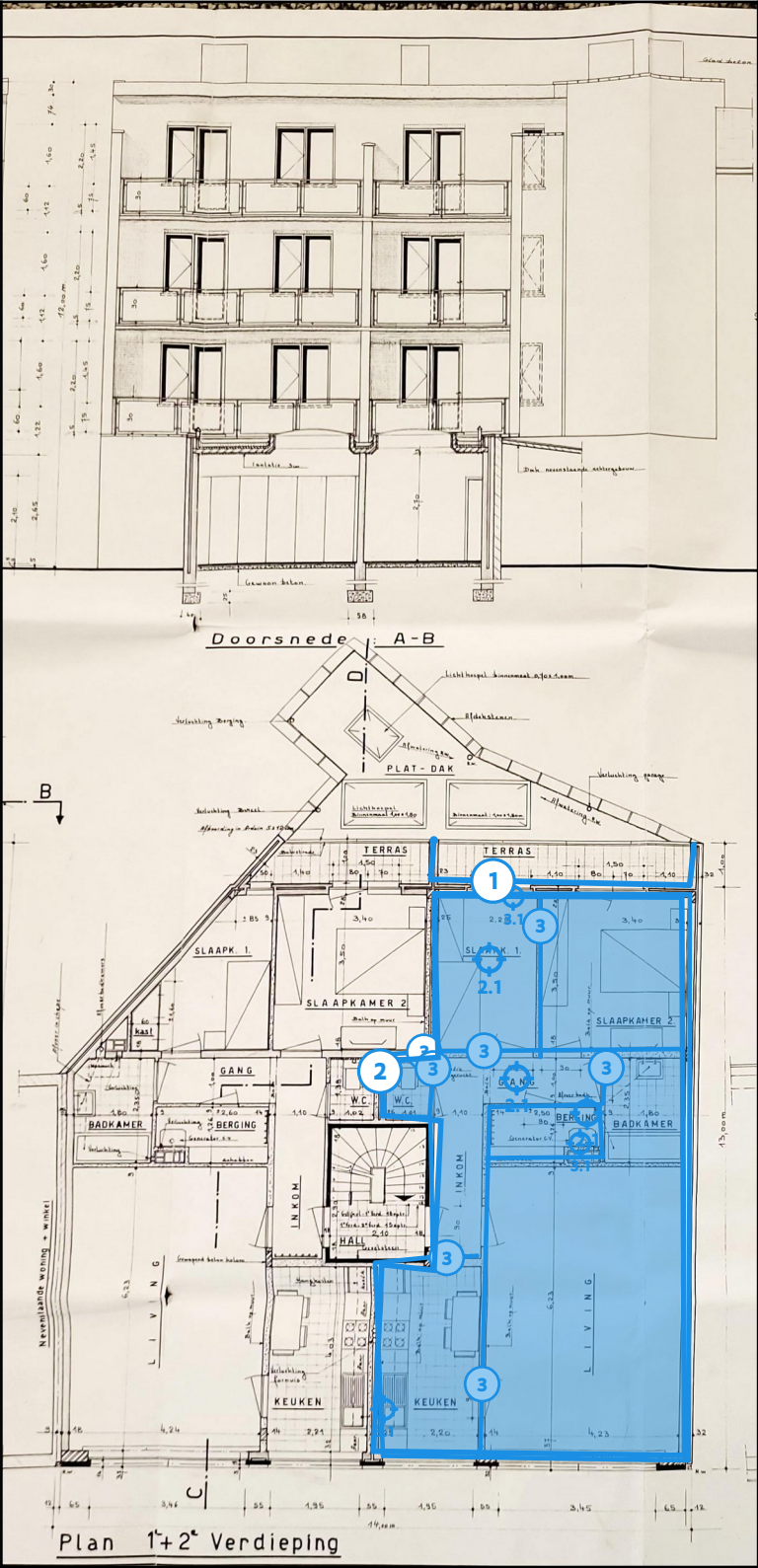
Legende van plan 1.1: Plan verdieping 1
