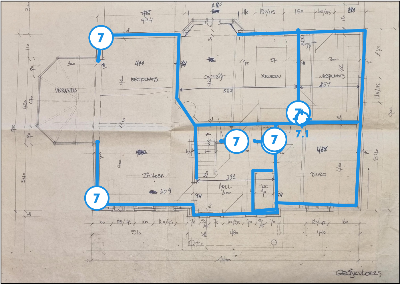
Legende van plan 1.1: Gelijksvloers (muren)
