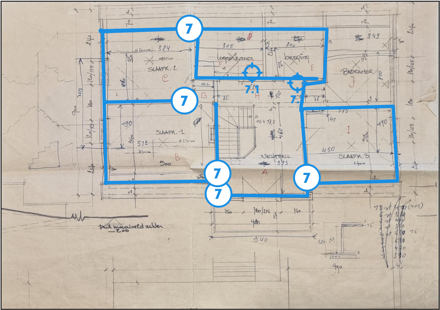
Legende van plan 1.3: Verdiep +1 (muren)
