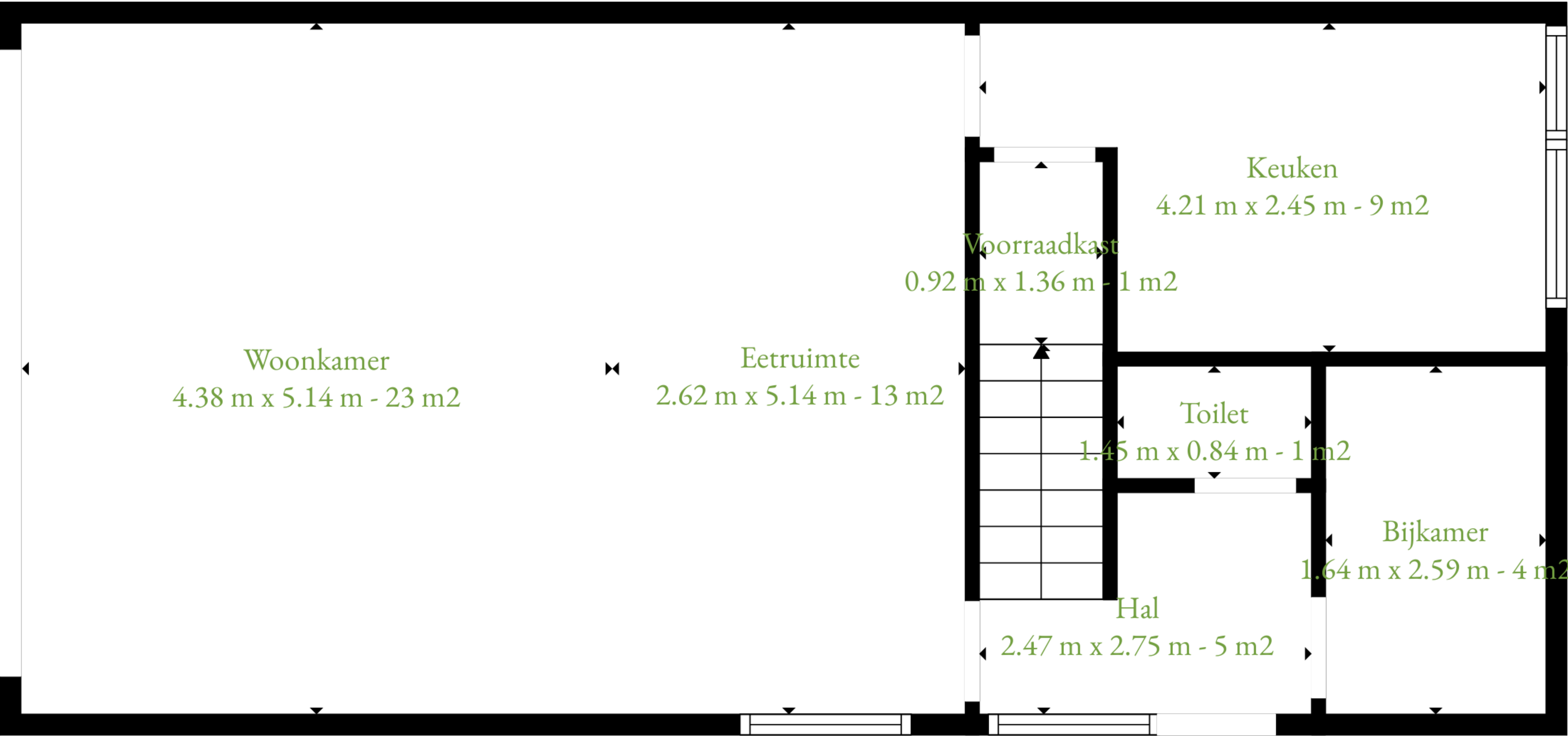
2. Verdieping
