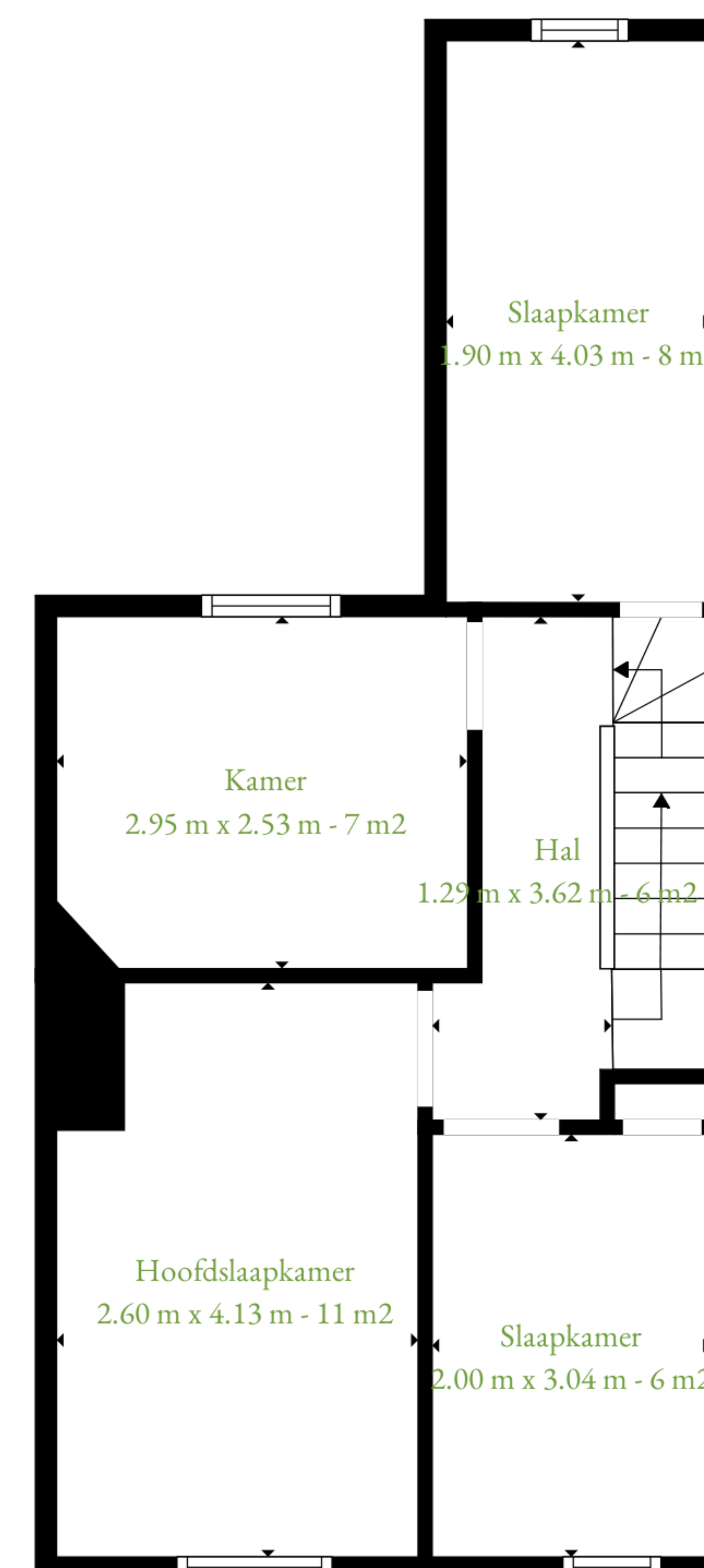
3. Verdieping
