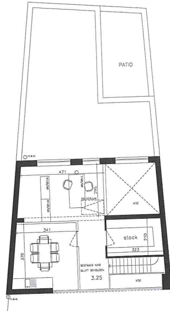
VERDIEPING
