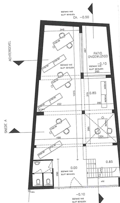
GELIJKVLOERS
