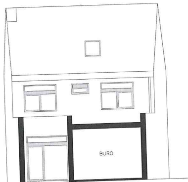
ACHTERGEVEL ONGEWIJZIGD
