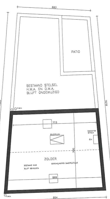
ZOLDERPLAN ONGEWIJZIGD
