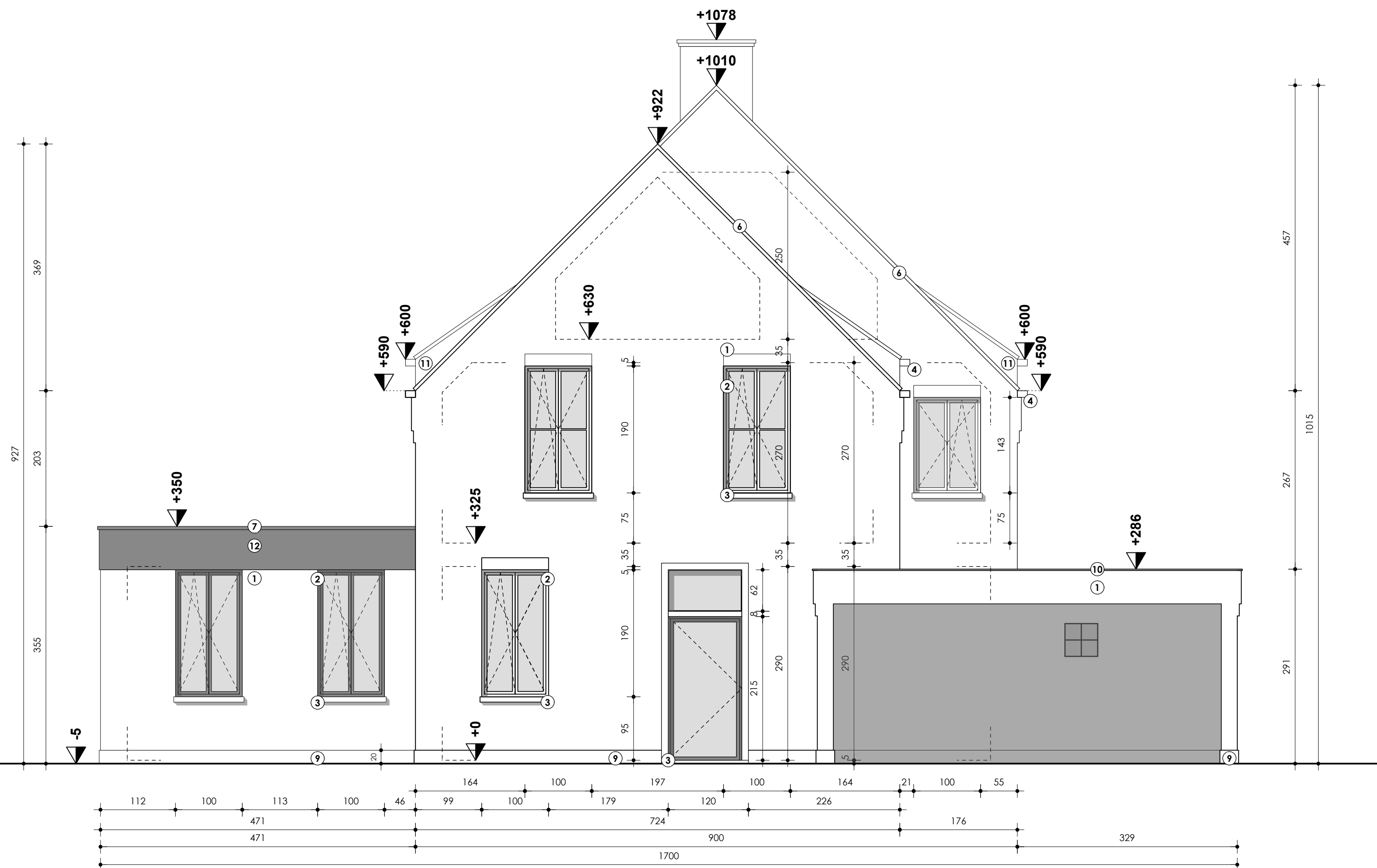
zijgevel links 1/50
