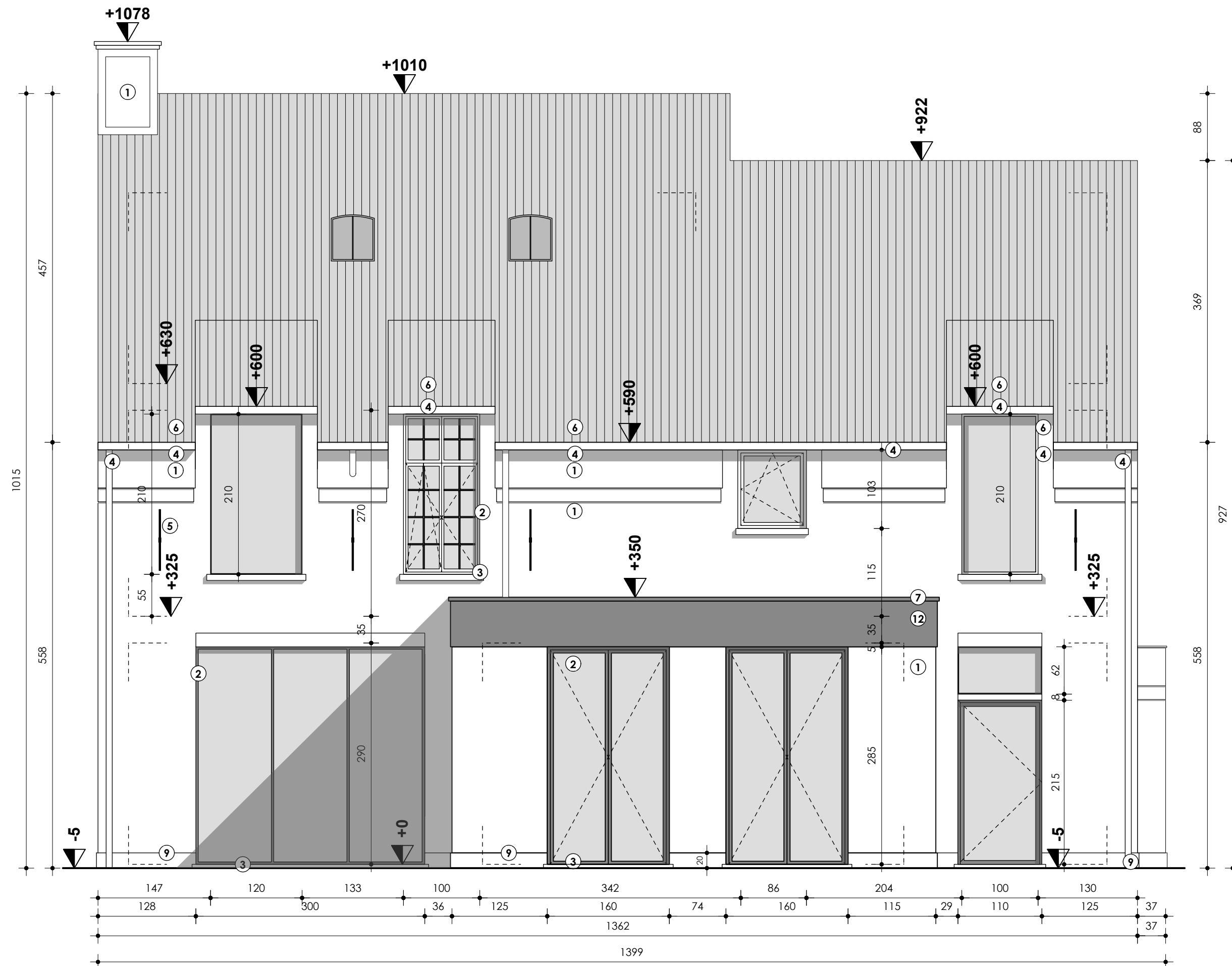
achtergevel 1/50
