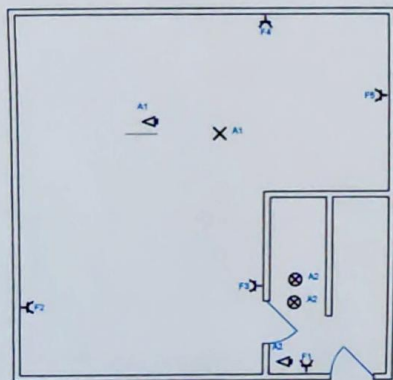
gelijkvloers garage
