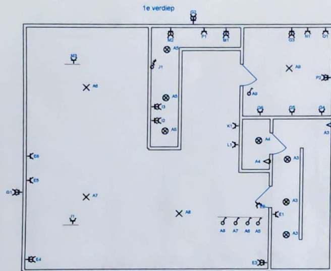
1e verdiep
