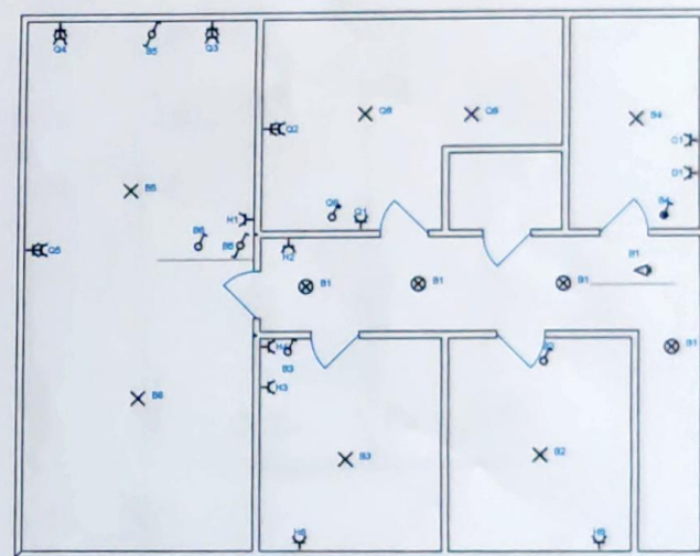
2e verdiep
