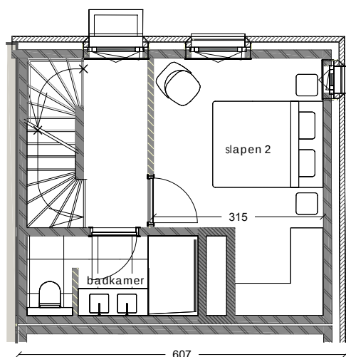
verdieping 1
