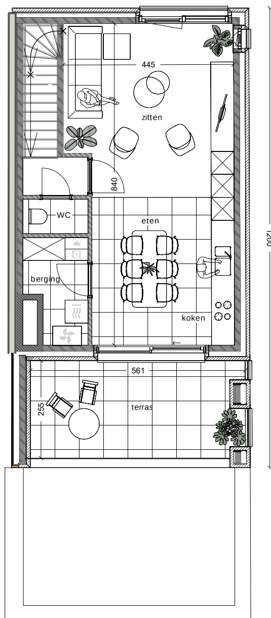
verdieping 2
