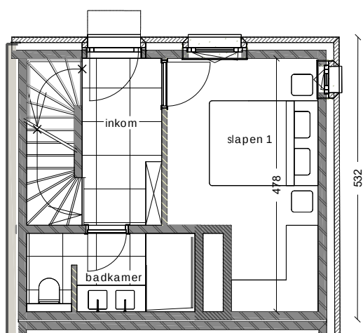
gelijkvloers
