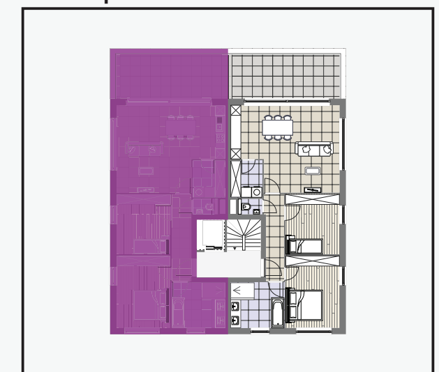
Grondplan
