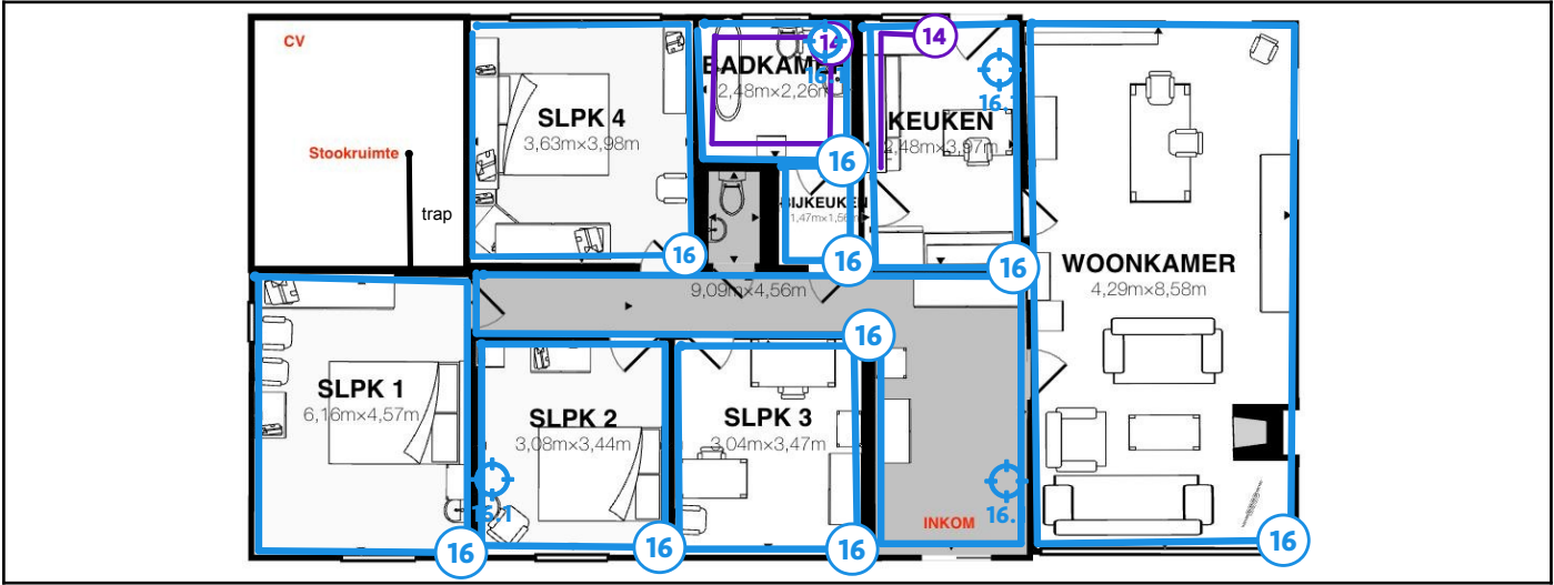
Legende van plan 1.2: Gelijkvloers (wanden)
