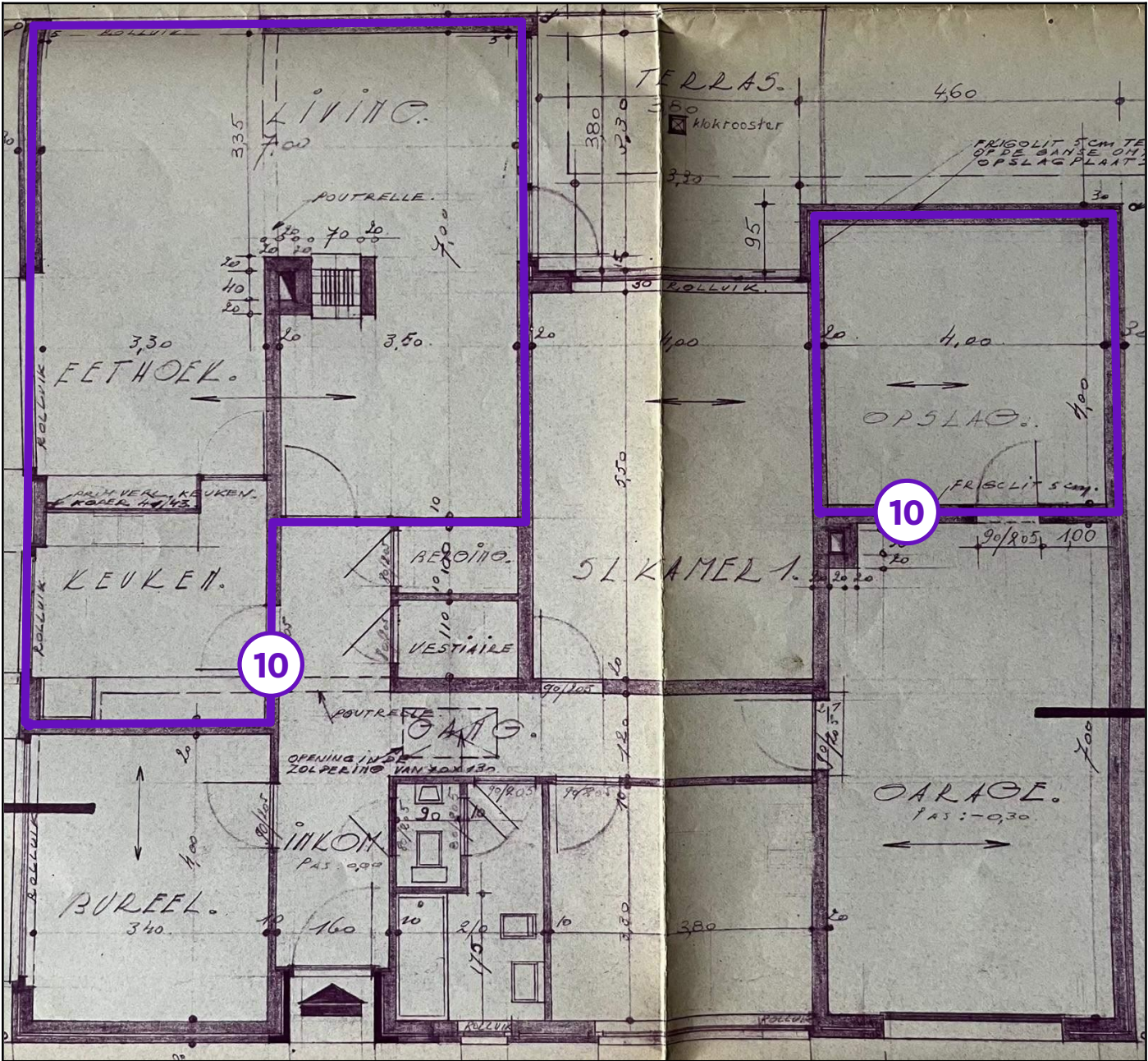
Legende van plan 1.2: Niveau 0 - plafonds
