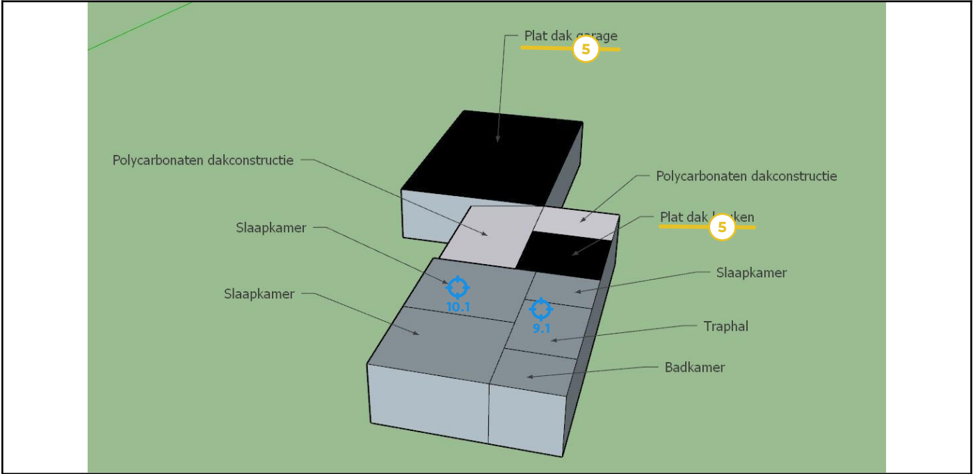
Legende van plan 1.3: Plan 1e verdieping
