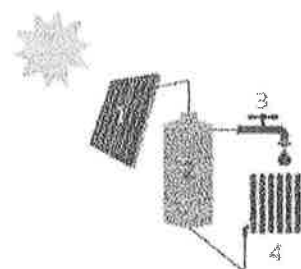
1. Zonnecollector | 2. Opslagvat zonneboiler | 3. Sanitair warm water | 4. Afgifta-element voor ruimteverwarming (optioneel)
