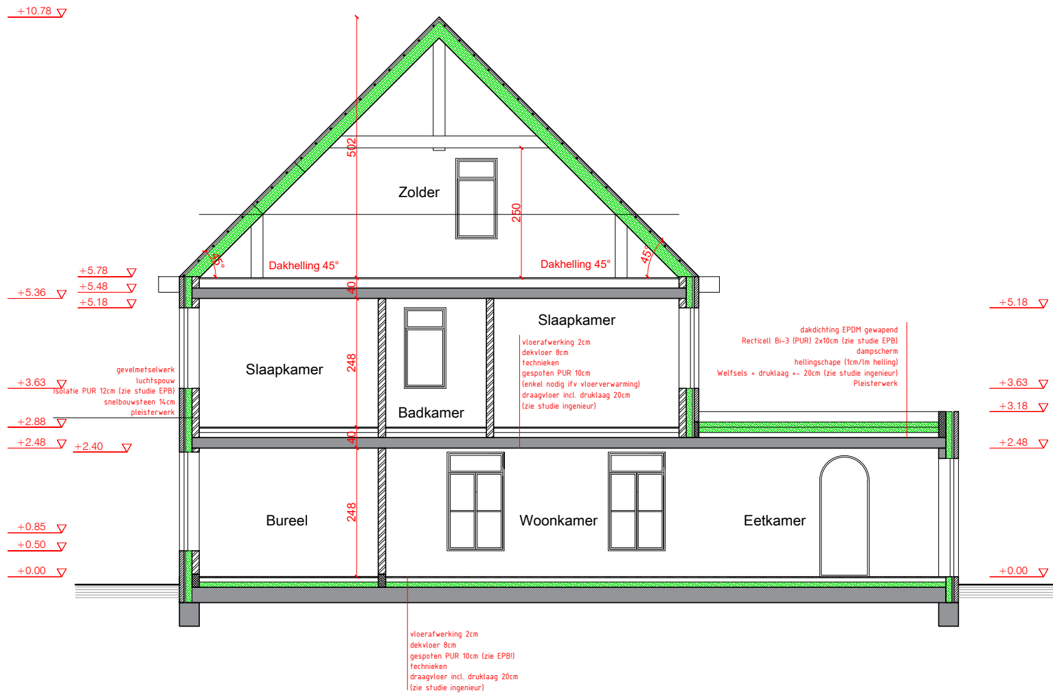
Snede A-A - 1/100
