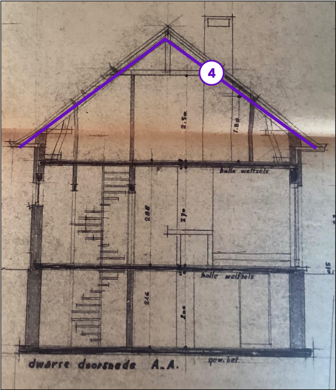
Legende van plan 1.6: Doorsnede
