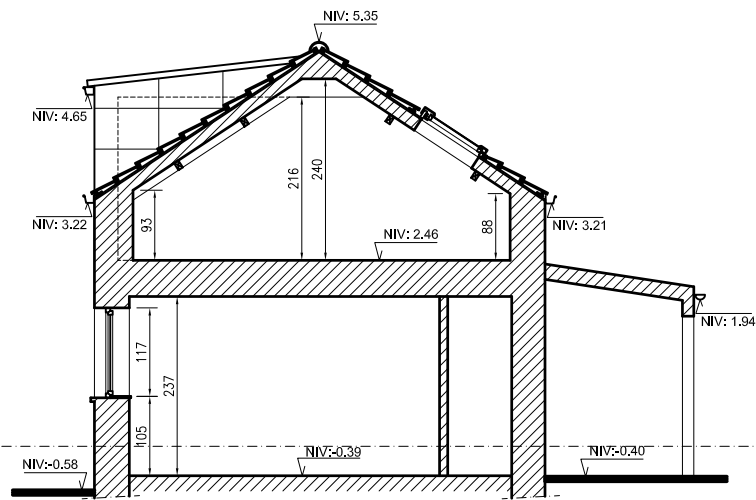
COUPE CC
