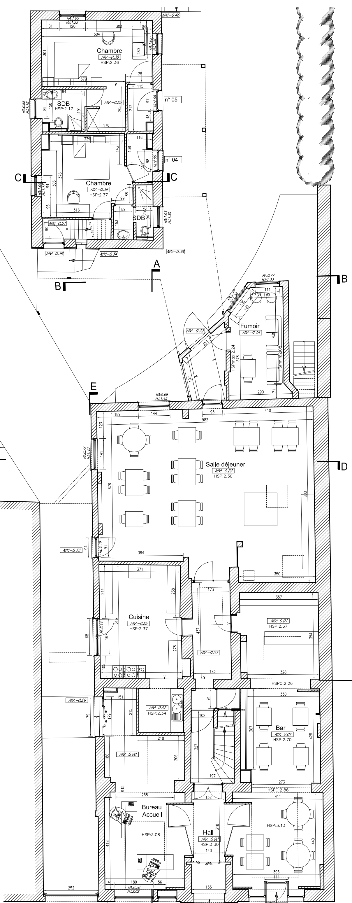
REZ DE CHAUSSEE
