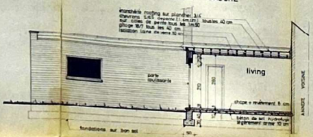
COUPE AB
