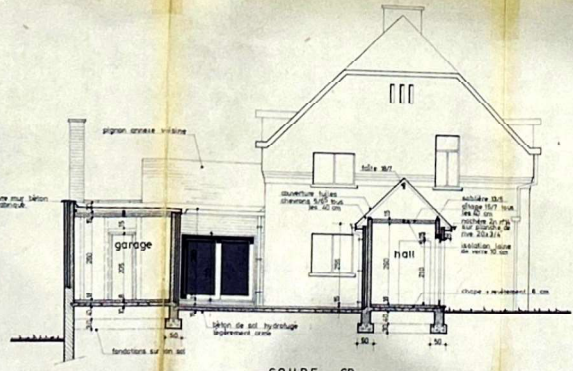
COUPE CD
