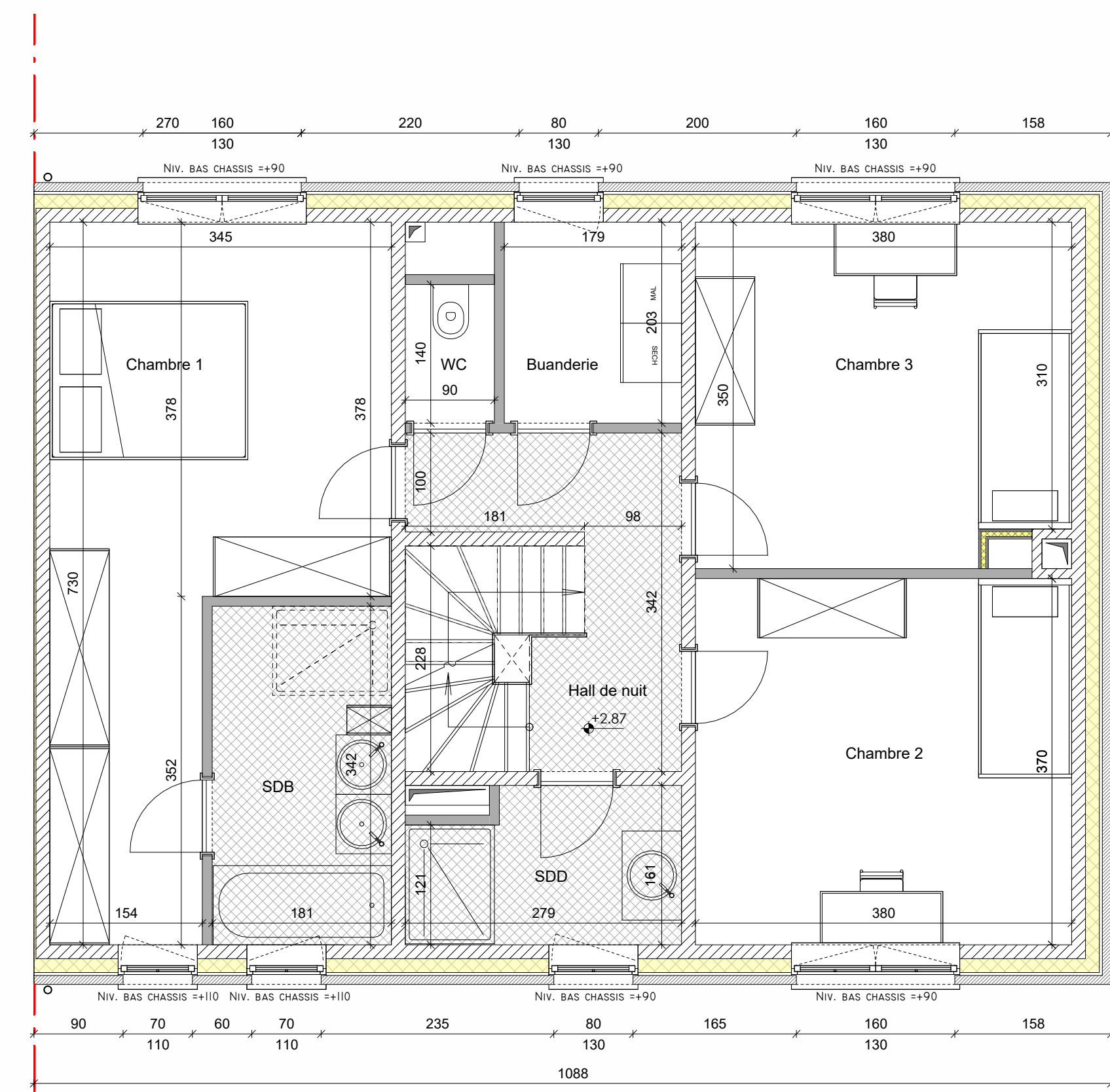
Premier Etage
