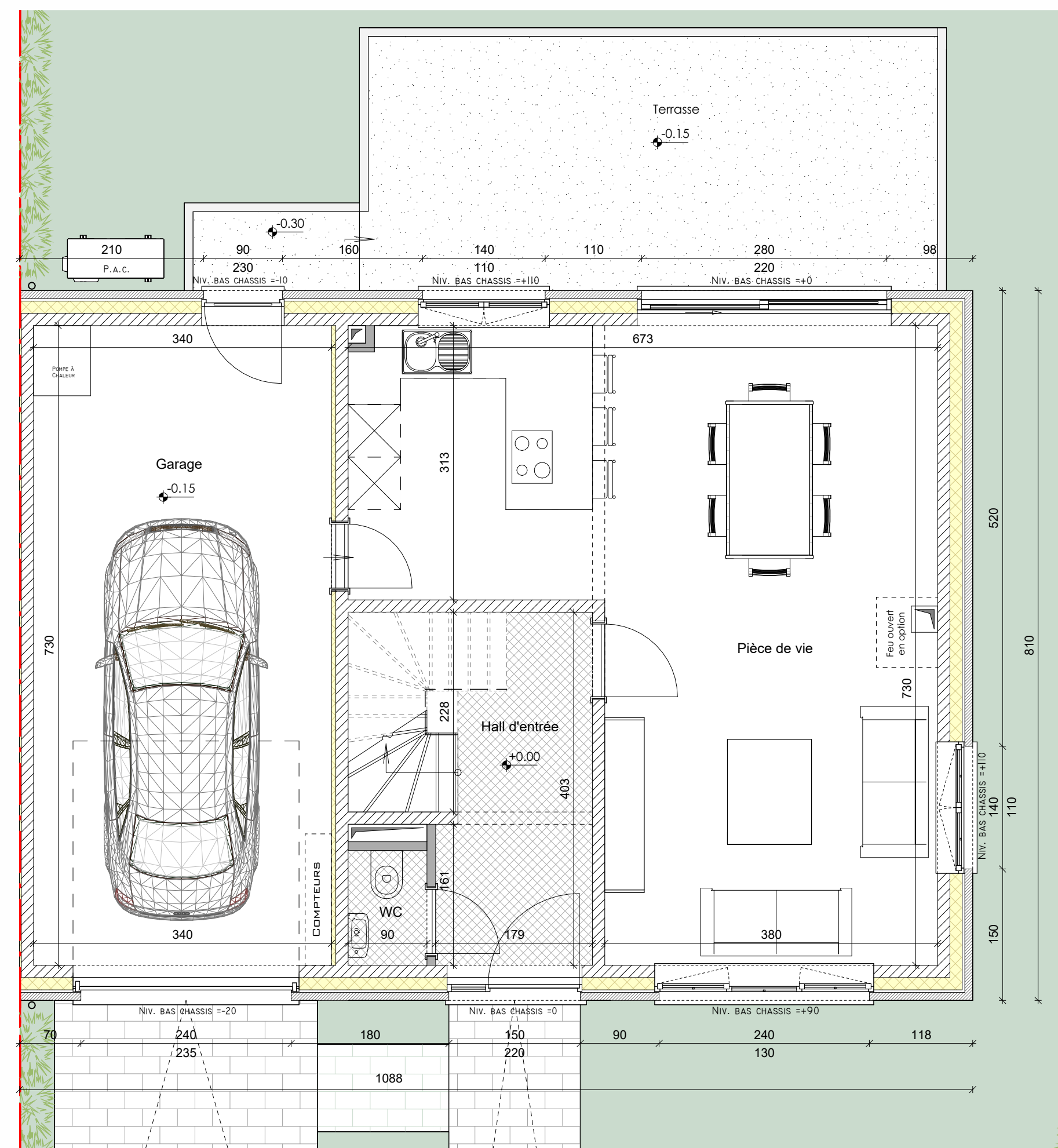
Rez-de-Chaussée
