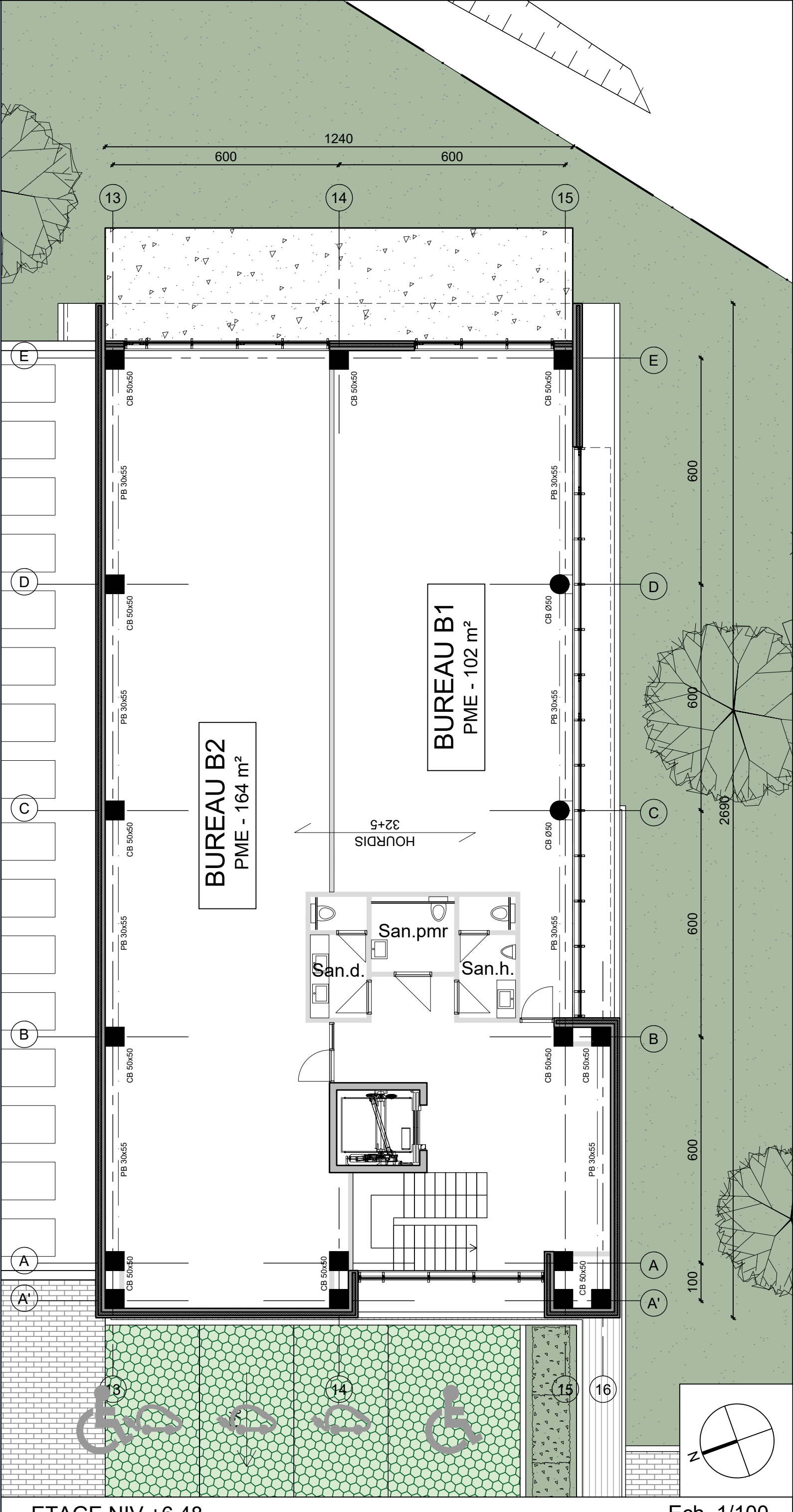
ETAGE NIV. +6.48 Ech. 1/100
