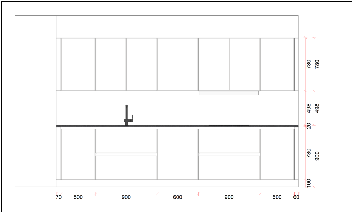
Elévation 2:
