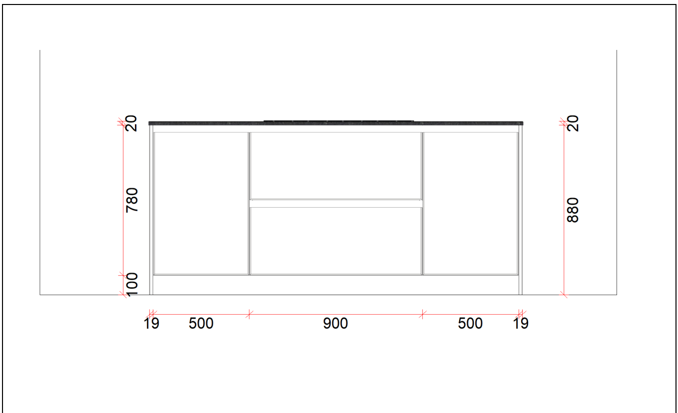
Elévation 2:
