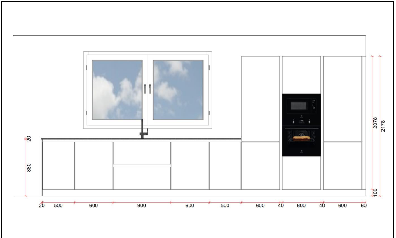
Elévation 1:
