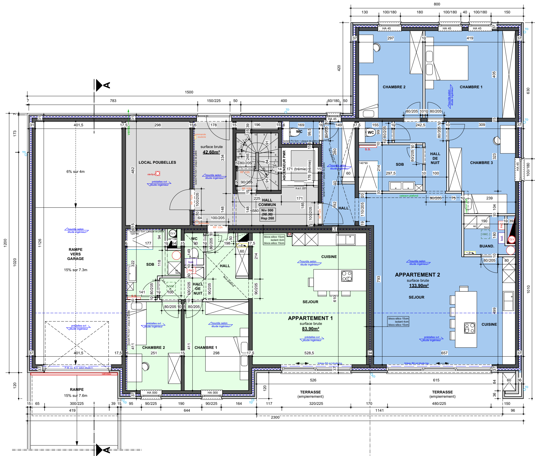
REZ-DE-CHAUSSEE (immeuble 2)
