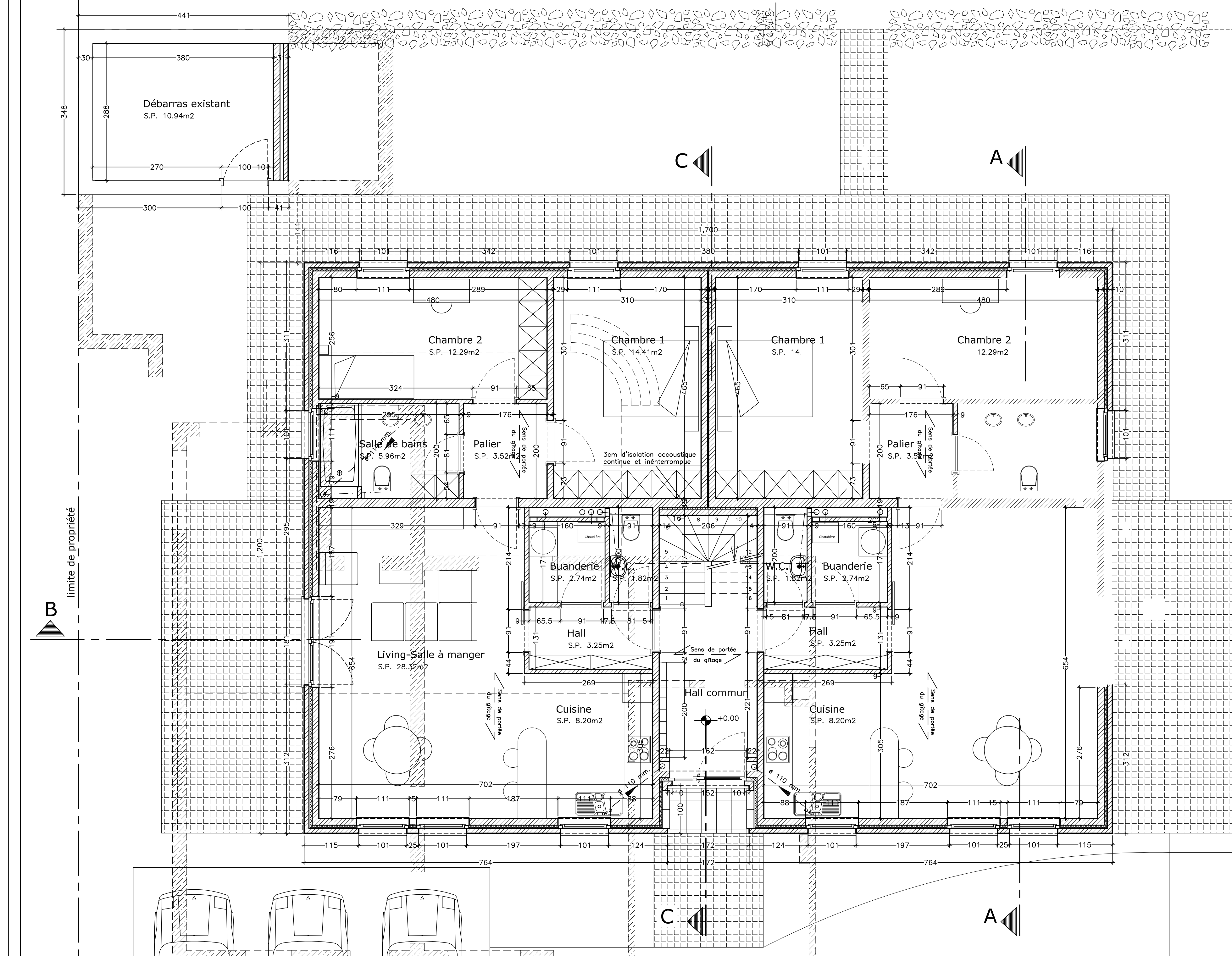
Rez-de-chaussée
