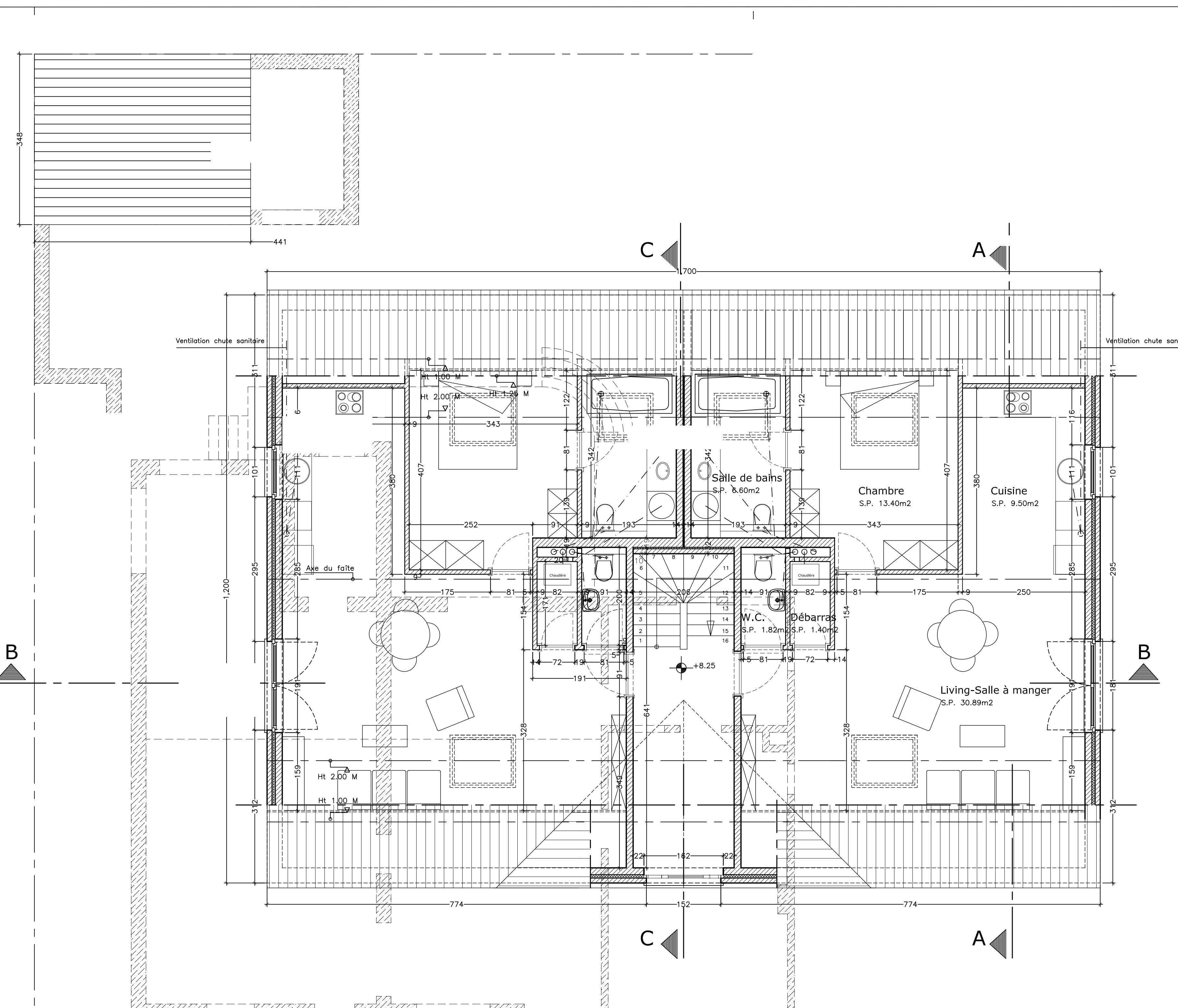
2ème étage
