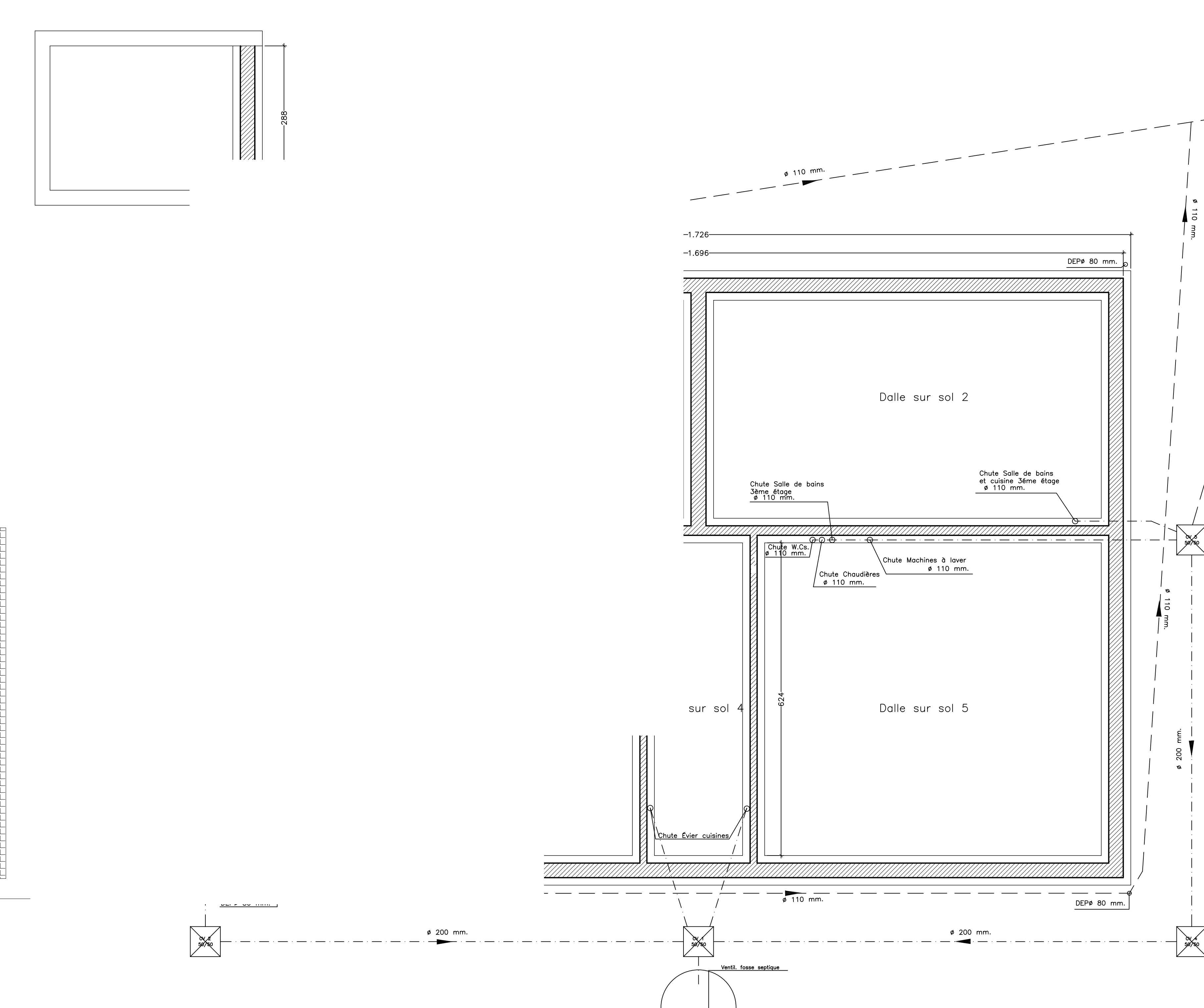
Fondations
