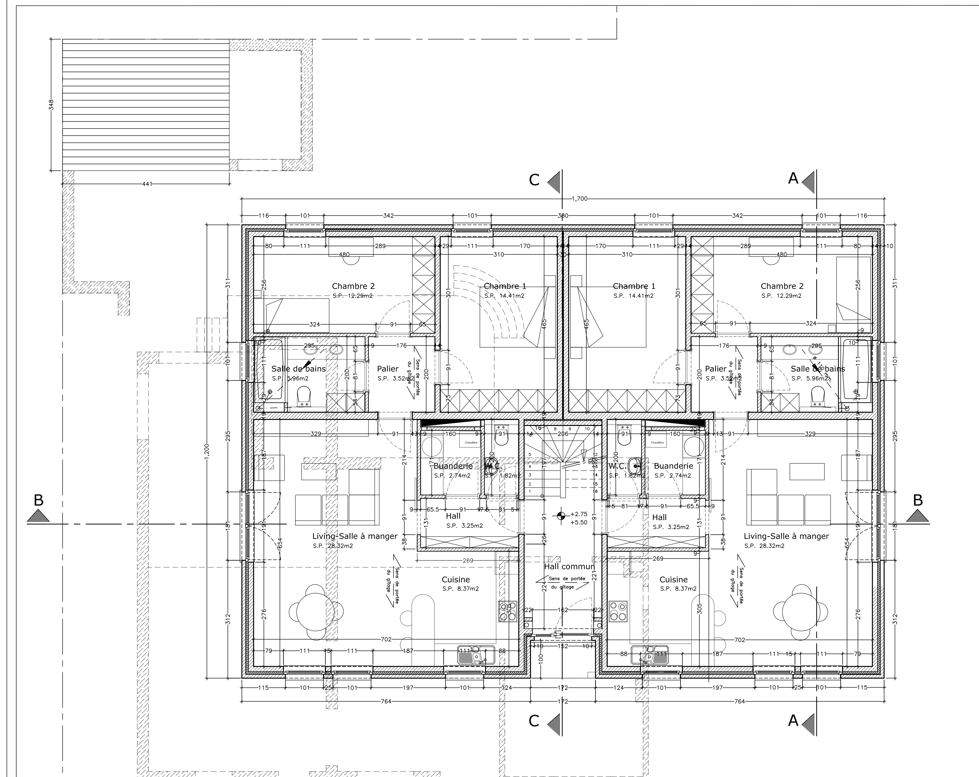
1er étage
