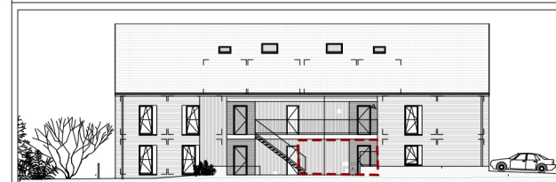
ELEVATION NORD-OUEST
