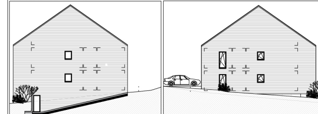
ELEVATION NORD-EST
