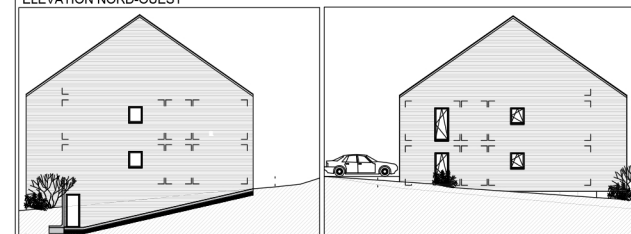
ELEVATION NORD-EST
