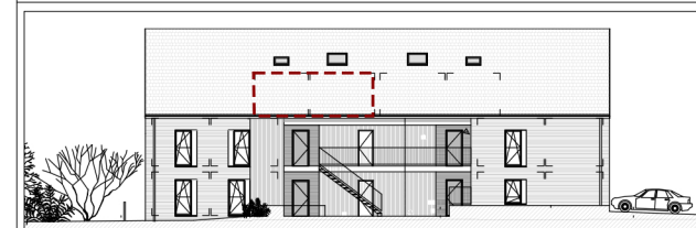
ELEVATION NORD-OUEST
