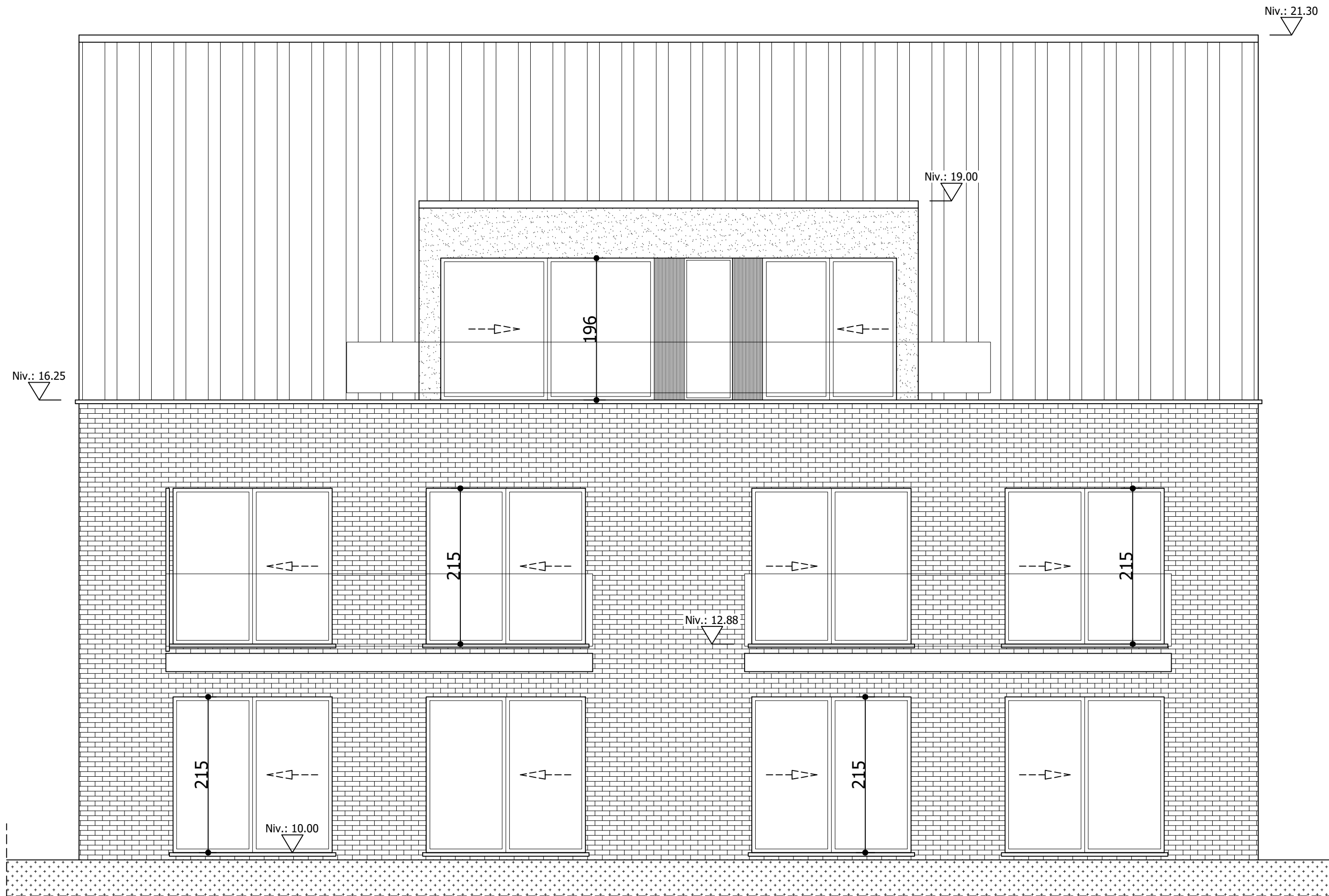
ELEVATION SUD-EST
