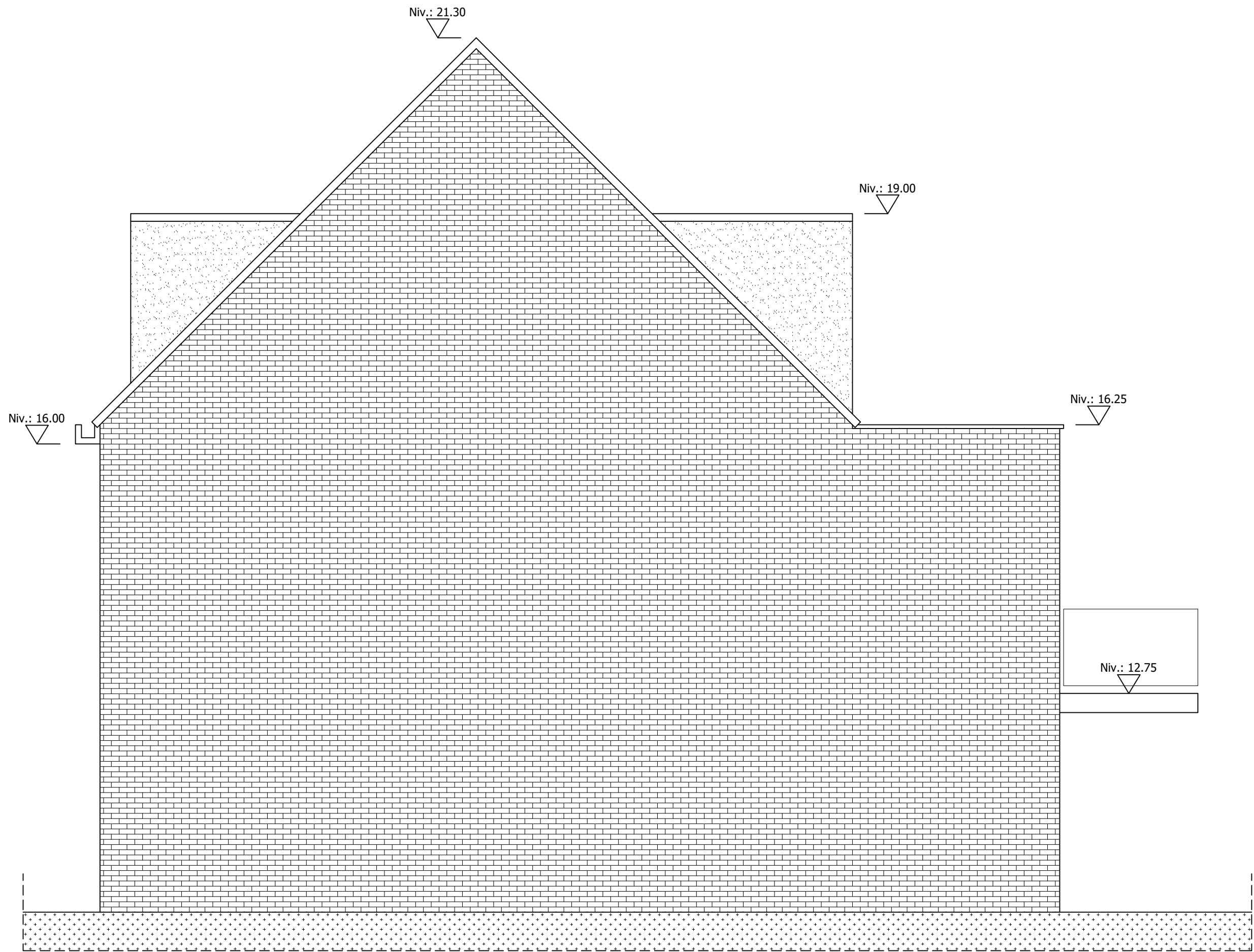
ELEVATION NORD-EST/ SUD-OUEST
