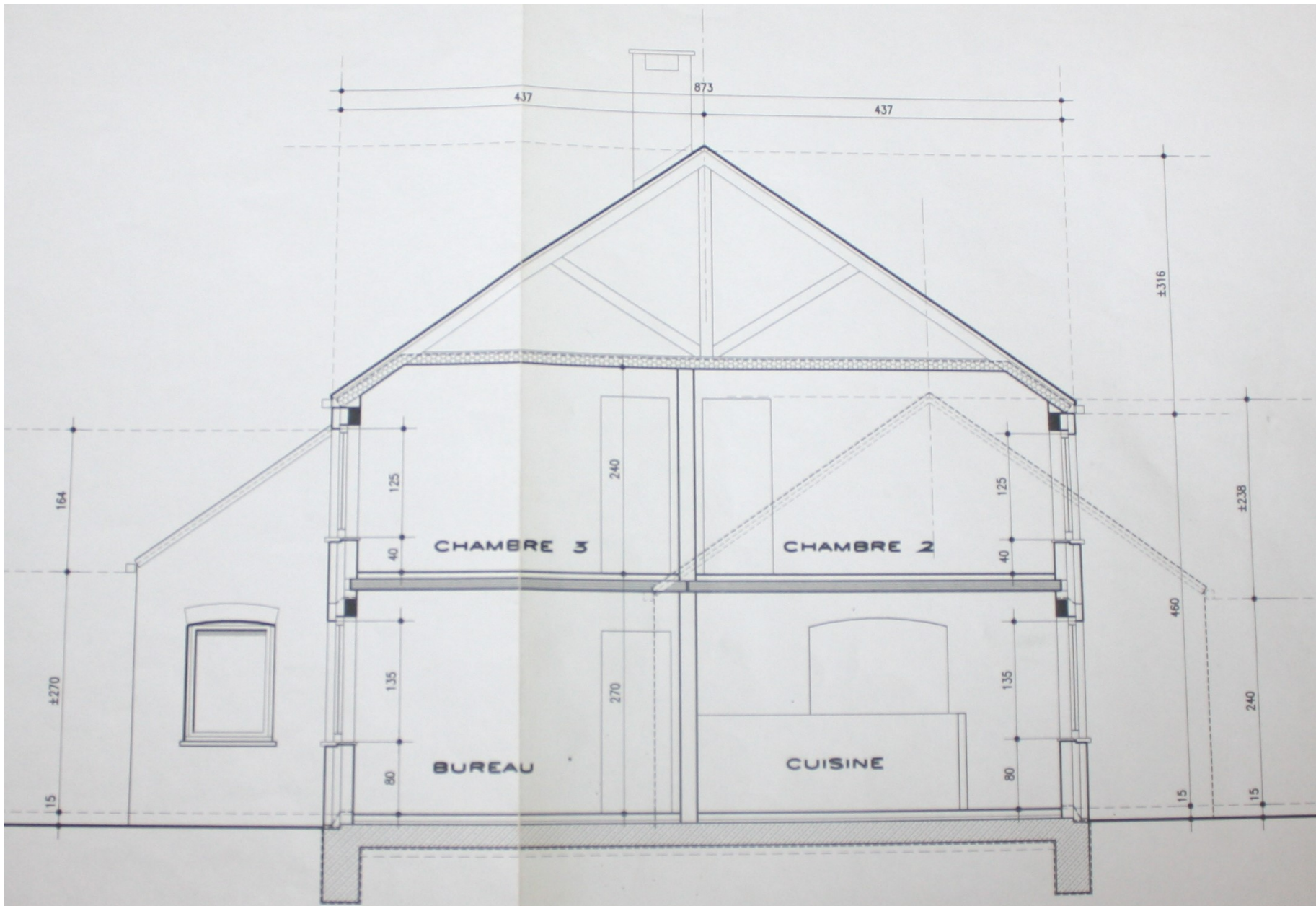
COUPE TRANSVERSALE
