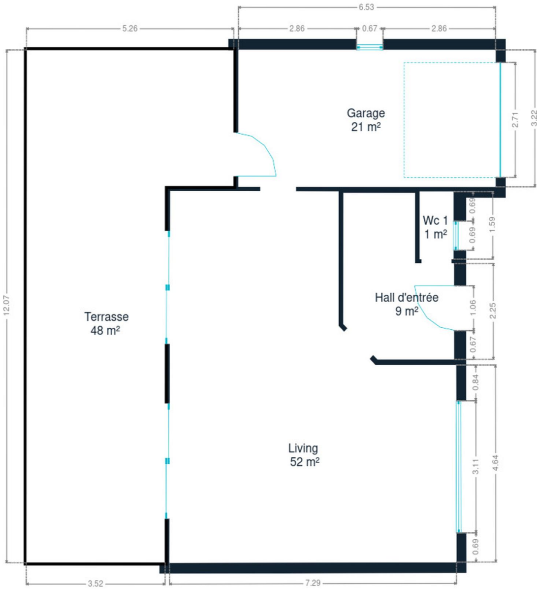
Rez-de-chaussée
