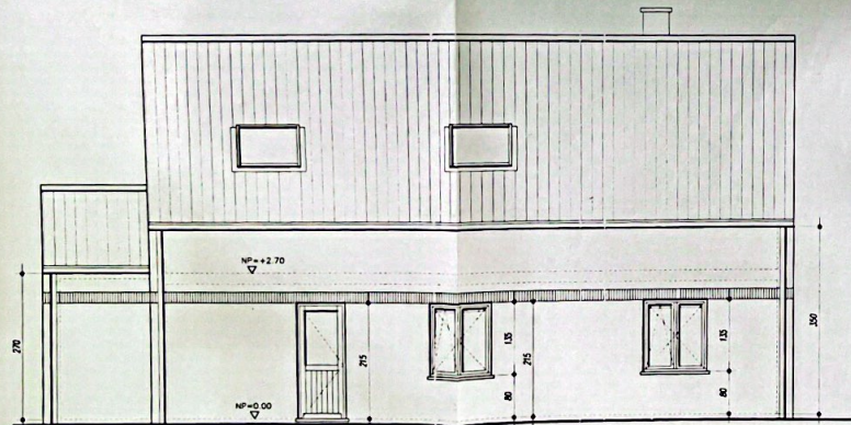
FACADE DROITE Ech. 1/50
