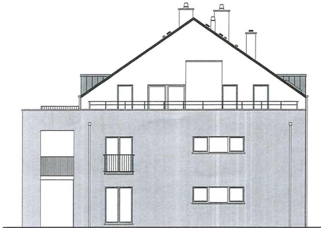
PIGNON AVANT
