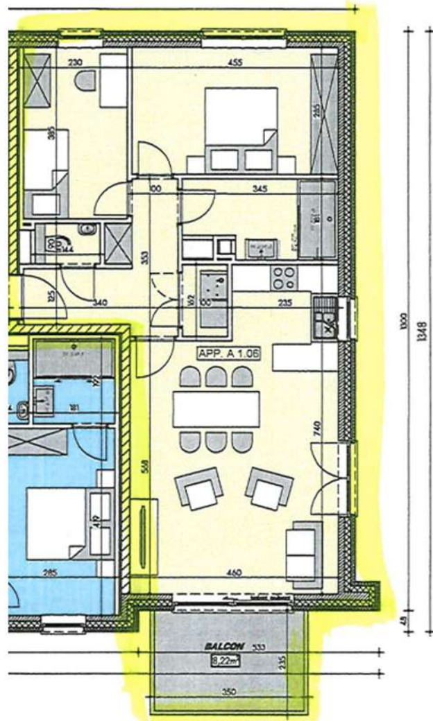
PLAN ETAGE
