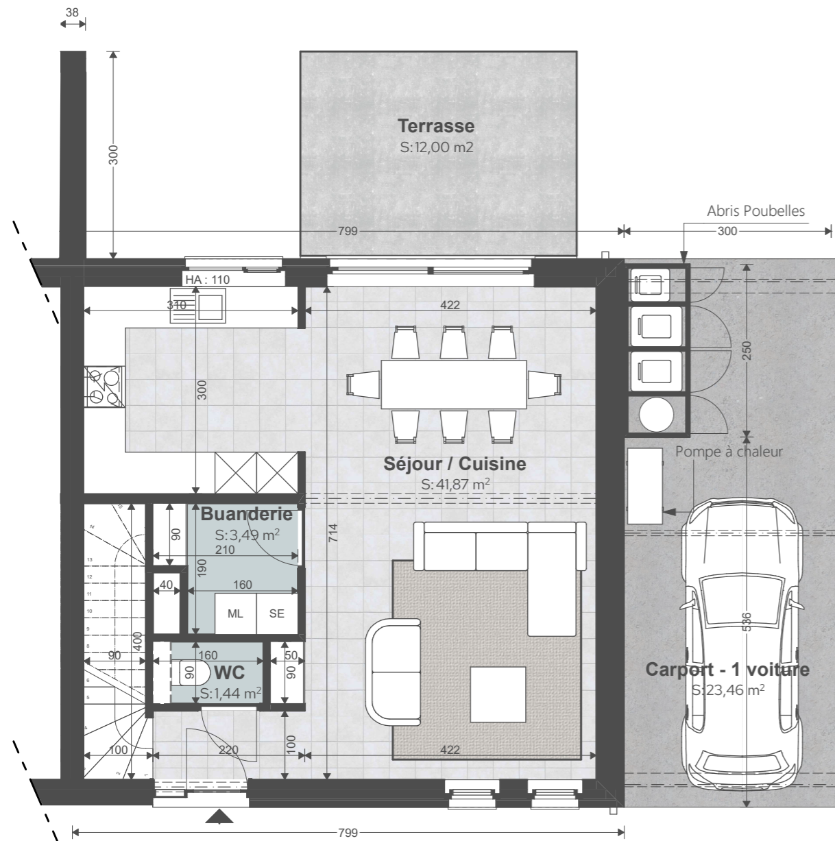
Rez-de-chaussée
