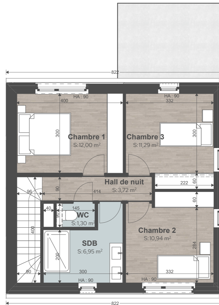
1er étage
