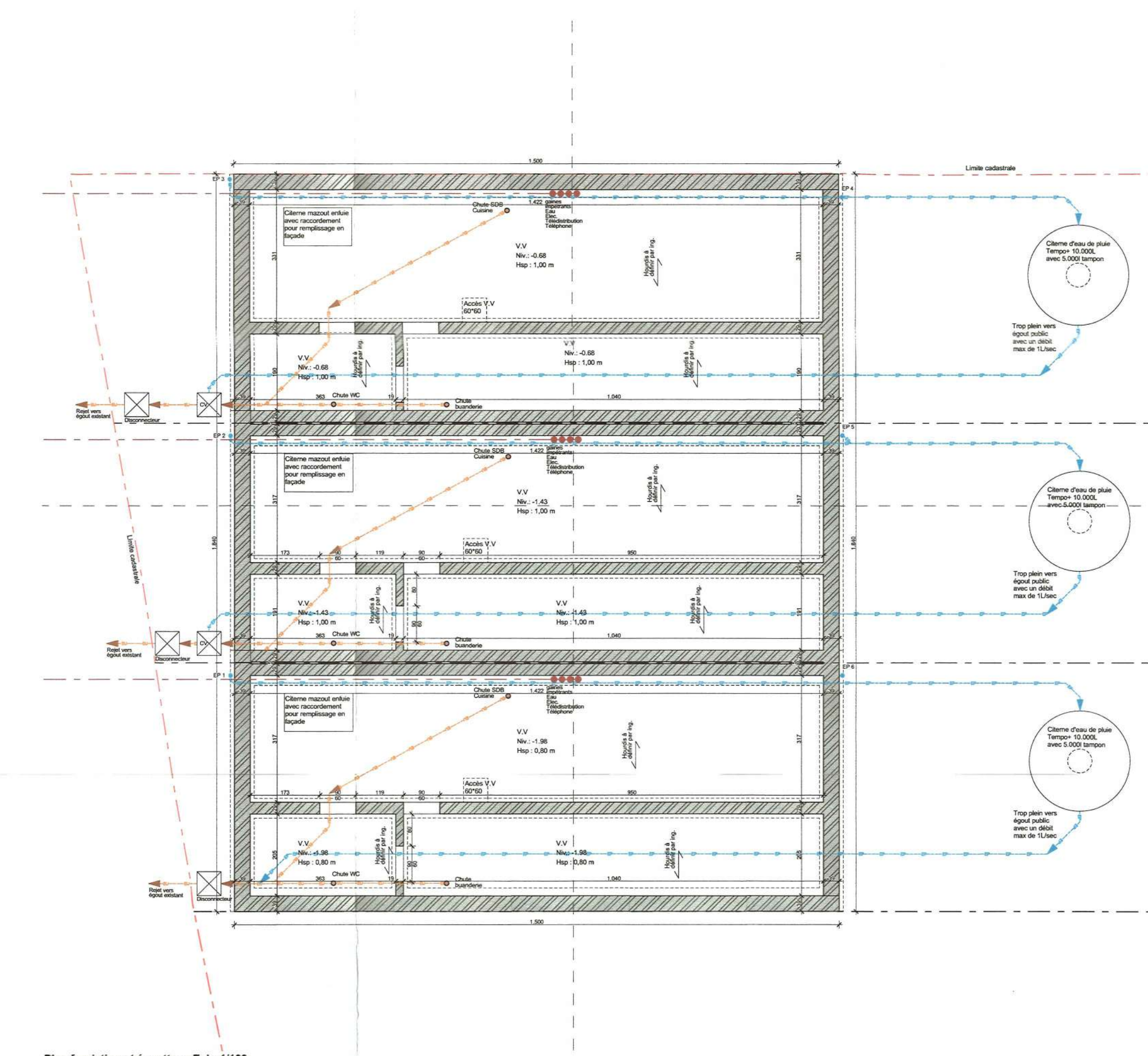
Plan fondation et égouttage Ech: 1/100
