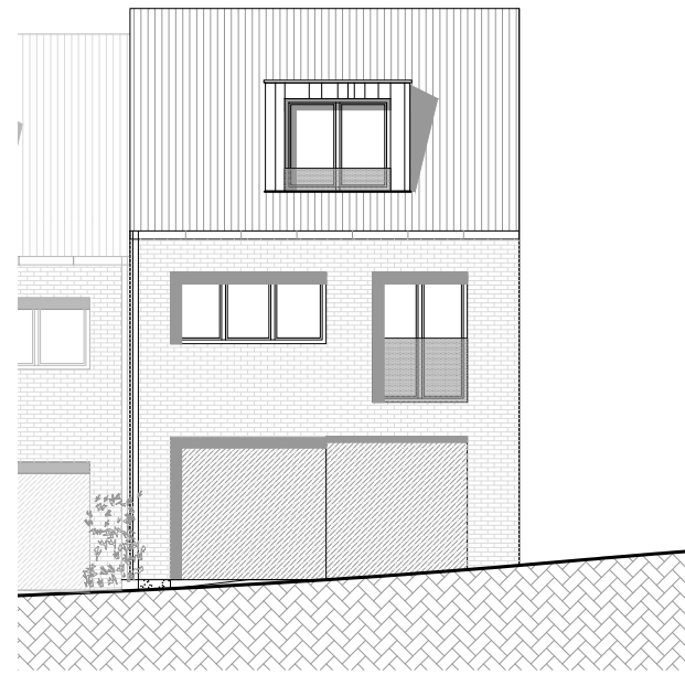
FACADE AVANT
