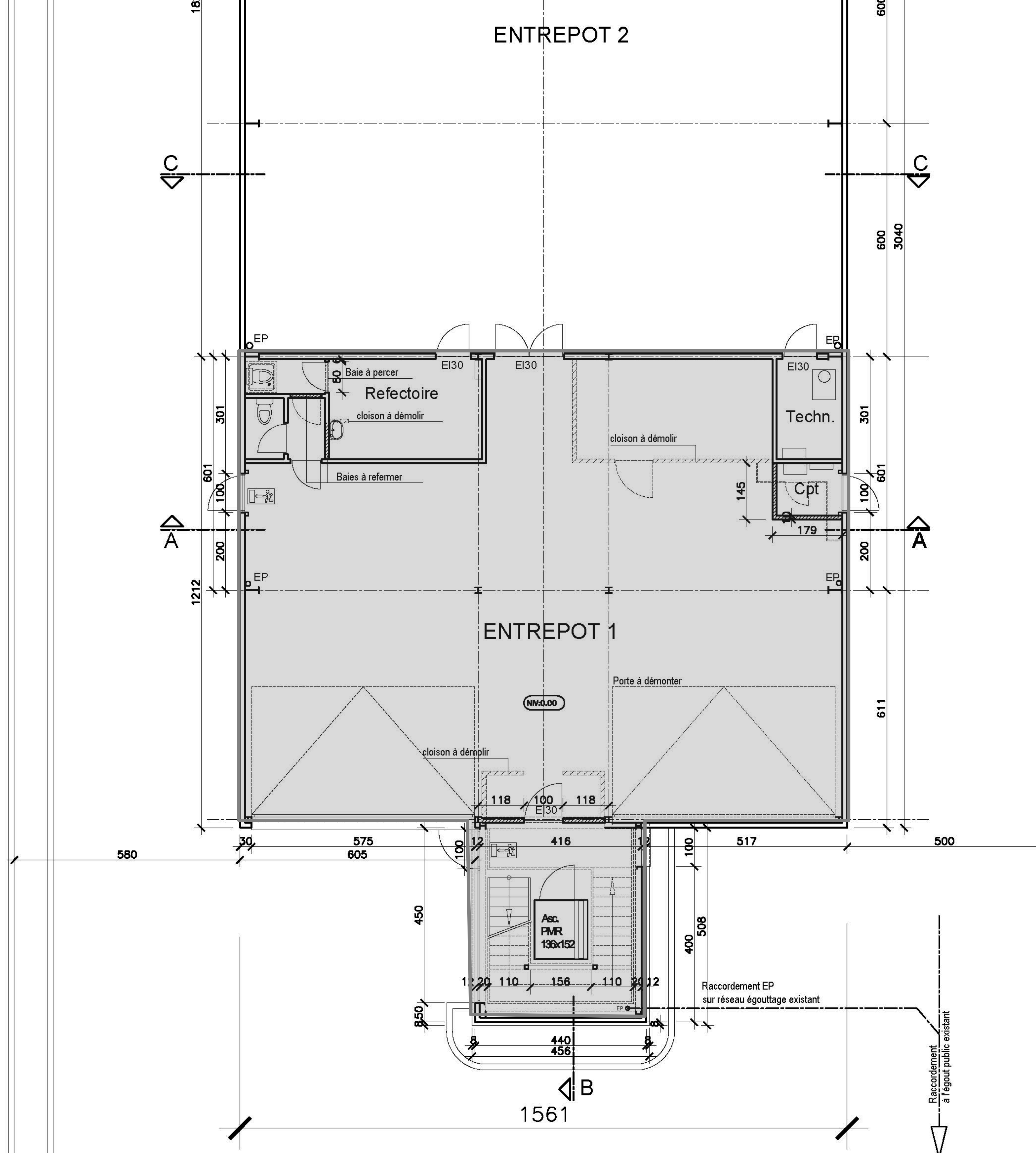
REZ-DE-CHAUSSEE
