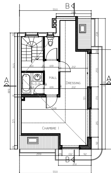
ETAGE SOUS TOITURE
