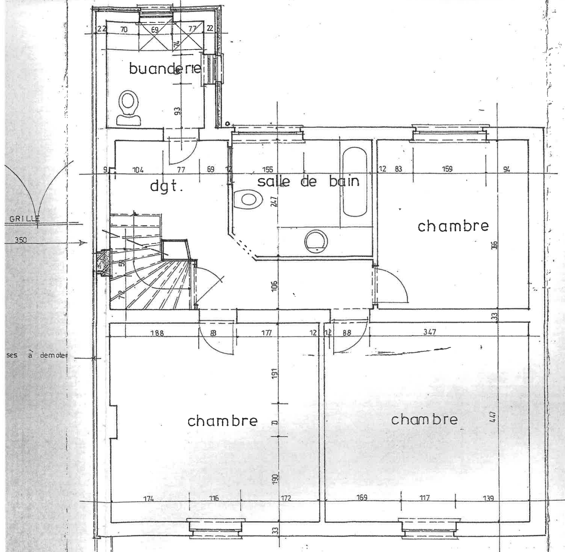
PLAN DE L'ETAGE
