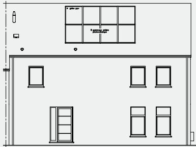
Façade avant
